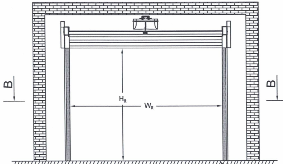
KÍCH THƯỚC KIỂM TRA ĐỂ LẮP ĐẶT
