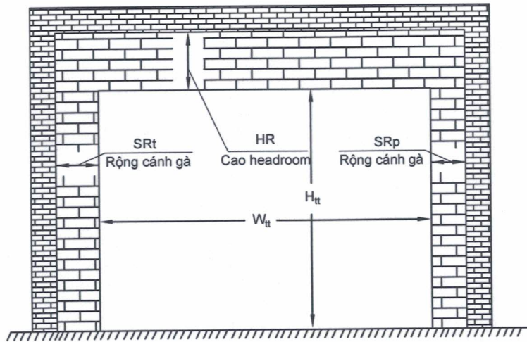
KÍCH THƯỚC KIỂM TRA ĐỂ LẮP ĐẶT
